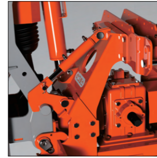
● 자동 유압 작동식 실린더 장착으로 폴딩 시 안정성 확보
