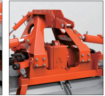
● 탑마스트 후방의 3점 hitch 장치 구비로 써레 등 부속 작업기 장착 용이
